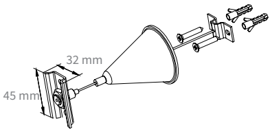
ovjesni komplet za tračne vodilice / suspension kit for track rail
